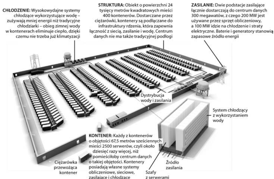
Rysunek 2.2. Rozszerzalne, modułowe centrum danych dla chmury. Warto zwrócić uwagę na brak zadaszenia. Kontenery z serwerami, zasilaniem, sprzętem chłodzącym i monitorującym mogą być dodawane i usuwane w miarę potrzeb. Źródło: magazyn „IEEE Spectrum”
